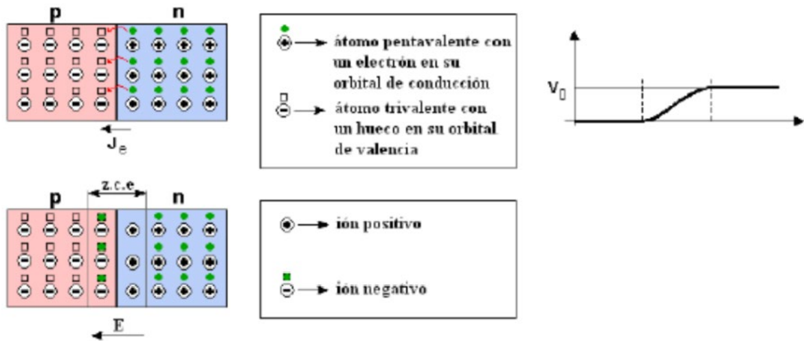
Figura 2: Unión p-n.
