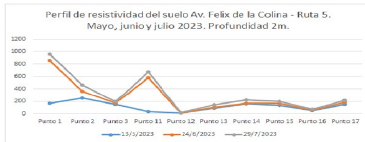
Figura N° 5.c: Perfil de Resistividad obtenidos en Avenida Félix de La Colina y Ruta Provincial N°5. Meses de mayo, junio y julio del 2023. Profundidades de 2m.
