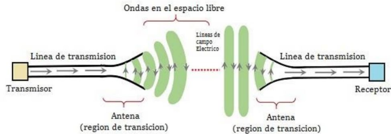
Figura 1: Esquema de antenas TX y RX
